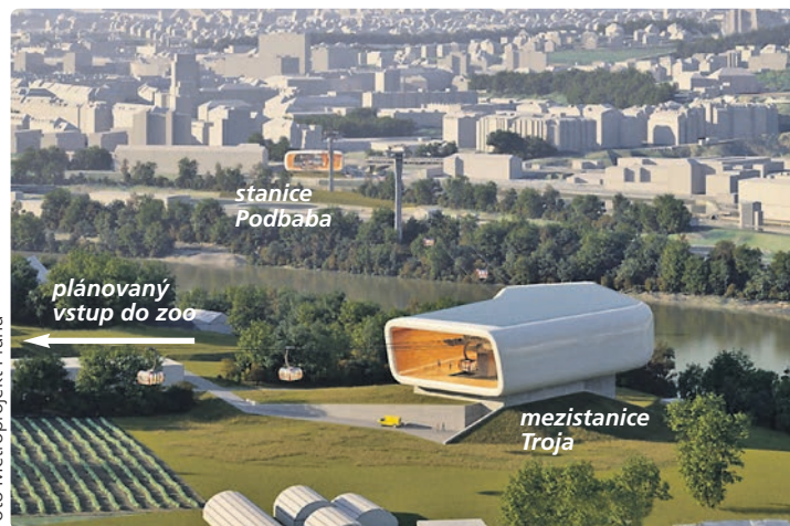
Vizualizace plánované lanovky Podbaba – Troja – Bohnice jsou čistě ilustrační a sloužily pro potřeby technické studie. Skutečná podoba stanic lanovky i sloupů vzejde teprve z mezinárodní architektonické soutěže.
