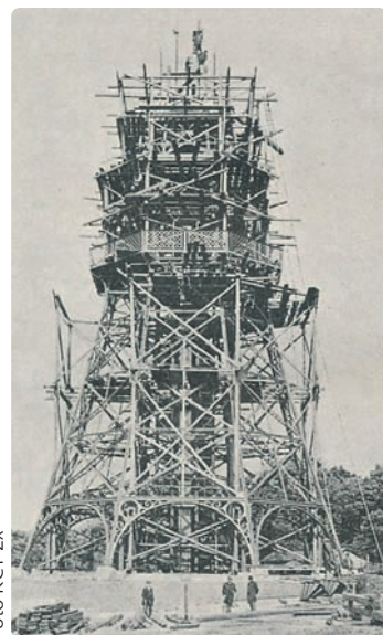
Rozhledna dosáhla 37 metrů, 13. června 1891
