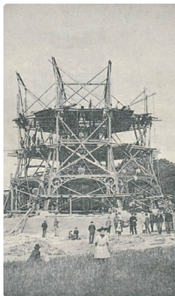
Rozhledna postavená po první patro, 27. května 1891
